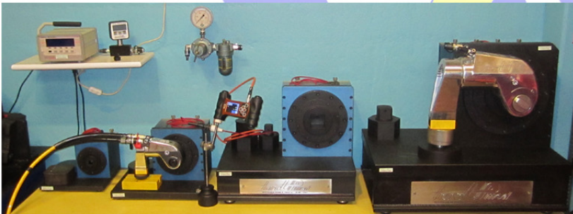
Banchi di Calibrazione Chiavi Idrauliche:
